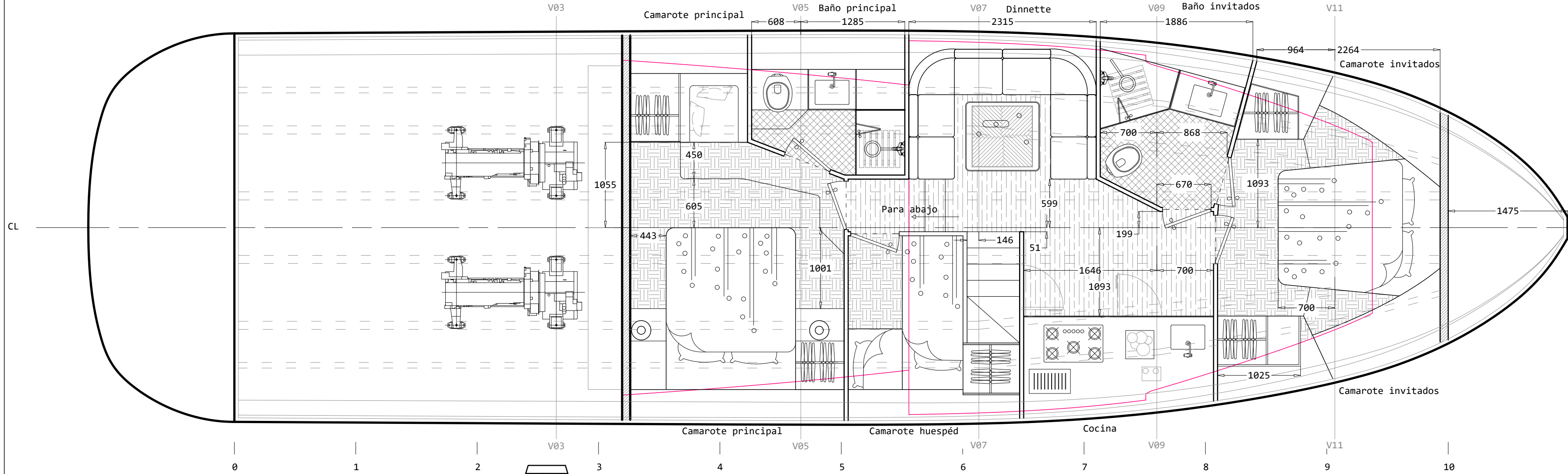
Piso 2: Camarotes
